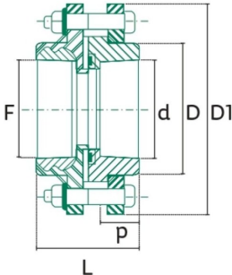
Plano Dimensional / Vista 2
